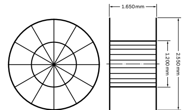
Abmessungen Stahlmehrwegtrommeln
