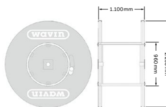
Abmessungen Einwegtrommeln aus Holz
