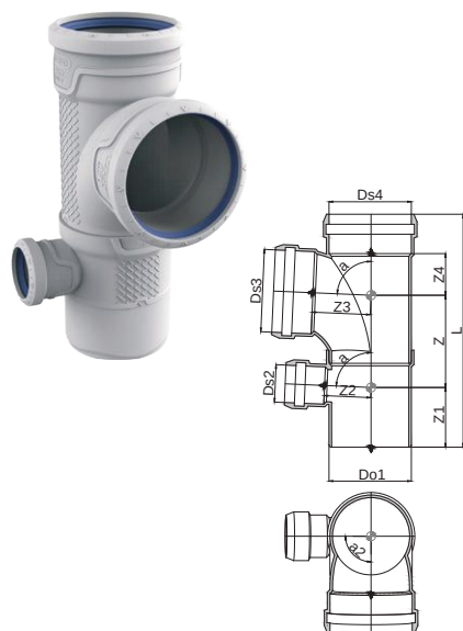
Wavin AS+ Duschdoppelabzweig > 87° > links
