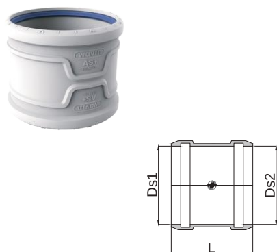
Wavin AS+ Überschiebmuffe
